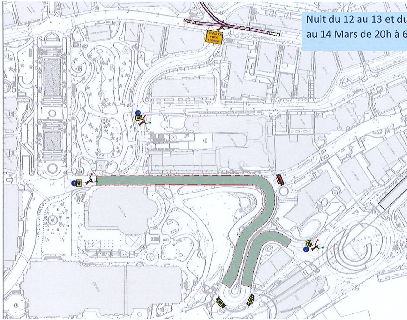
FIGURE 3 : PLAN D'INSTALLATION DE CHANTIER AV DES SPELUGUES
